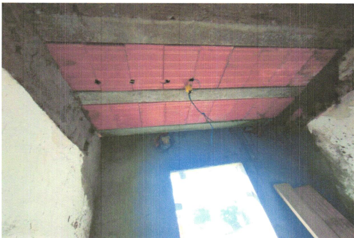
FOTO 07 - Laje pré-fabricada treliçada para piso ou cobertura, intereixo 38cm, h=12cm, el. enchimento em EPS h=8cm, inclusive escoramento em madeira e capeamento 4cm.2016
